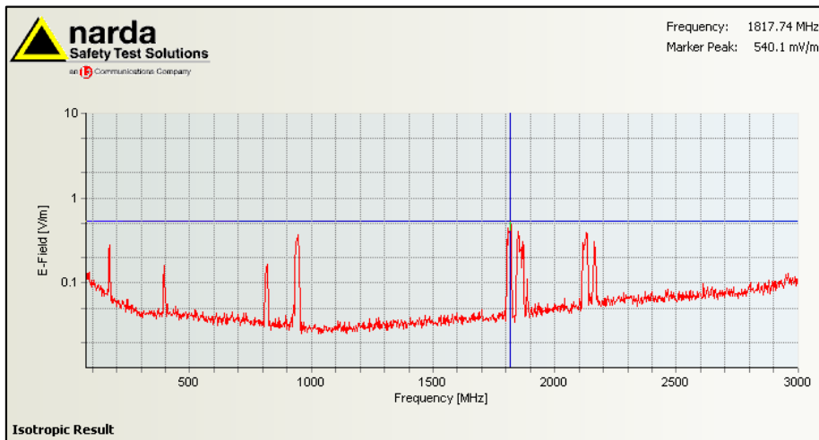
Figuur 1; Selectieve veldsterkte meting ingezoomd op sterkst aanwezige signaal, 1817.74 MHz, DCS (GSM1800).
