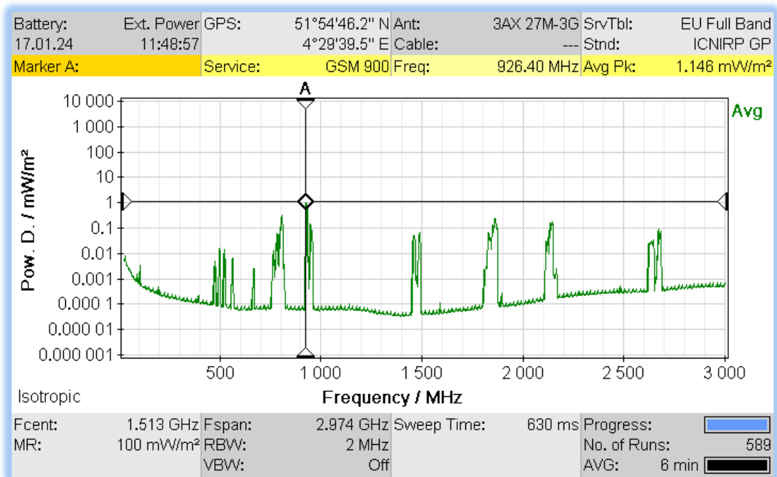
Figuur 7: Plot van de selectieve EMV-meting, in de keuken
