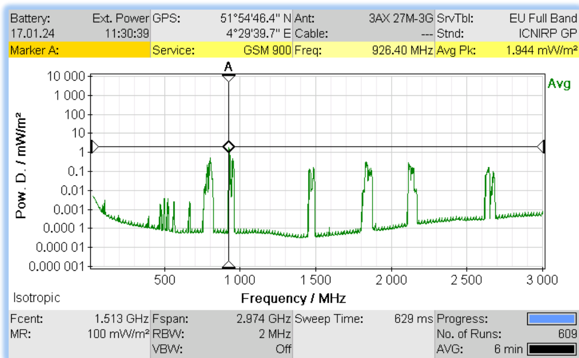
Figuur 6: Plot van de selectieve EMV-meting, op het balkon
